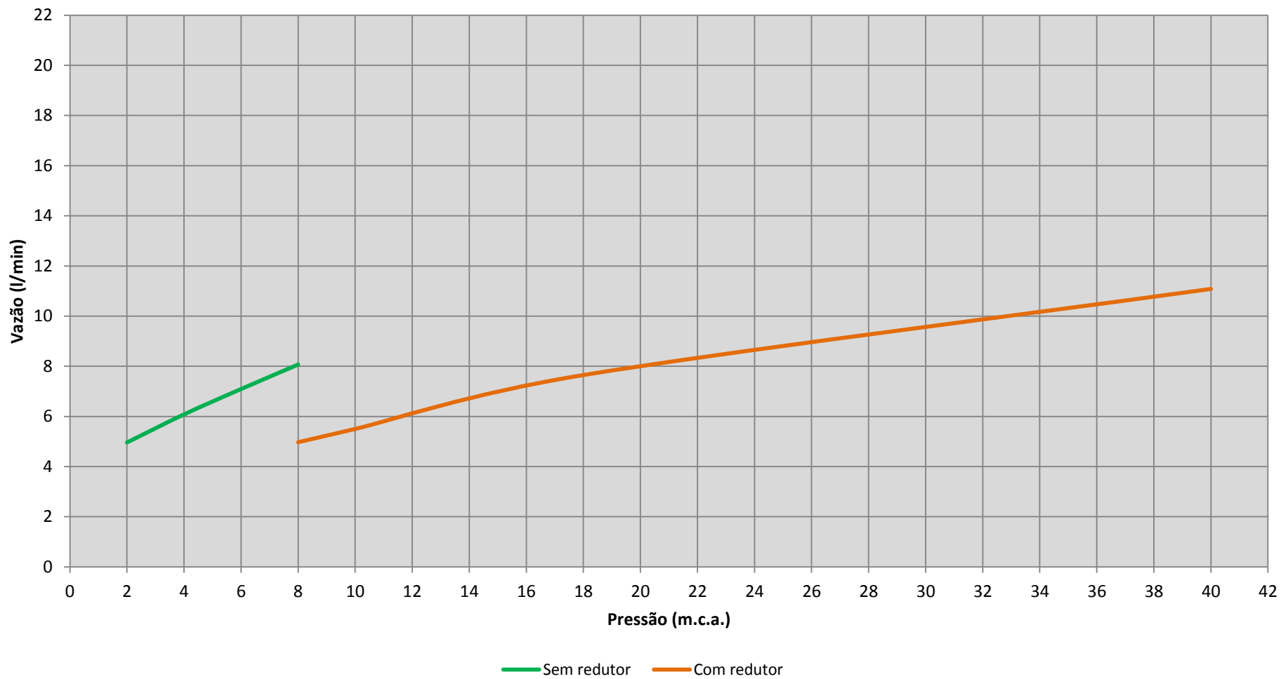
Curva de vazão - Ducha SS 3T
